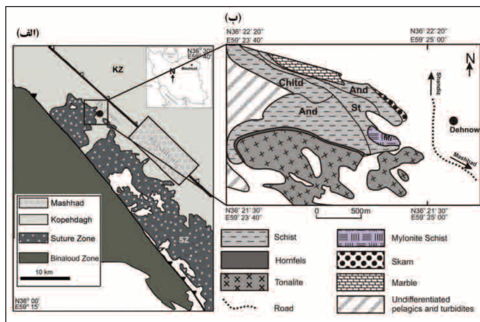
شکل ۱- نقشه زمین‌شناسی (الف) محدوده‌های ساختاری اصلی در شمال‌خاوری ایران (پس از Alavi, 1991)، ب) موقعیت منطقه مورد مطالعه در نقشه زمین‌شناسی ایران و نقشه زمین‌شناسی منطقه مورد مطالعه (اقتباس از نقشه زمین‌شناسی ۱/۱۰۰۰۰۰ طرجه، پورلطیفی، ۱۳۸۱).
