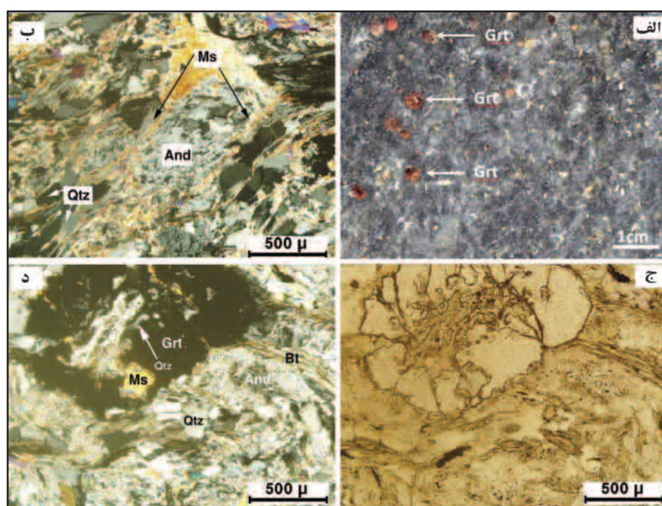
شکل ۲- (الف) نمایی از گارنت شیس کلریتویددار در نمونه دستی؛ (ب) گارنت در تصویر XPL؛ مسکوویت در اطراف بلورهای آندالوزیت؛ ج و د) ارتباط و حضور گارنت در کنار مسکوویت، بیوتیت و آندالوزیت در نمونه گارنت کلریتوید شیس و حضور میانبار مسکوویت و کوارتز درون گارنت.
